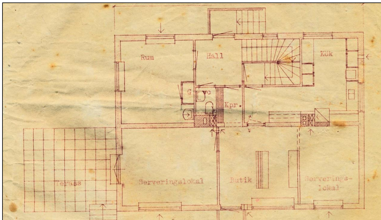
Ritning över entréplanet.
